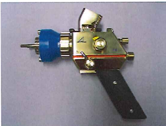
パウダー溶射ガン「ユニスプレージェット(USJ)」 ノズルアクセラレータ付
