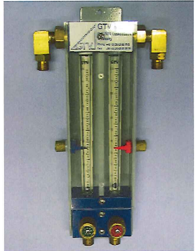
2GFタイプフローメーター(酸素/アセチレン) Flowmeter Type 2GF for O2 and Ace
