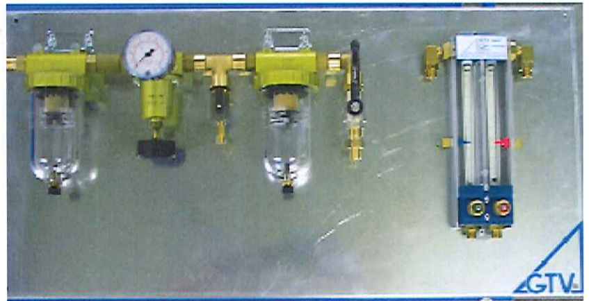
ガス/エア供給パーツ GAS and AIR Supply
