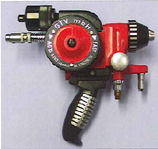
11Eタイプワイヤ溶射ガン Wire Flame Spray Gun Type 11E
