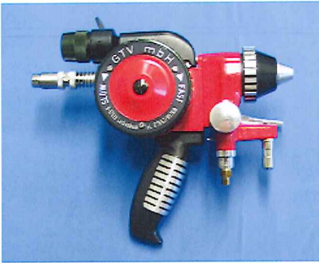
12Eタイプワイヤ溶射ガン Wire Flame Spray Gun Type 12E
